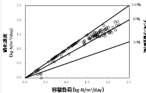
図1 硝化性能
