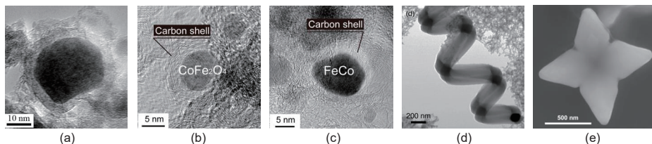
図 1 臨界流体中の自己集積化過程により形成されるナノ構造体。(a) フェロセン溶解二酸化炭素の光分解による鉄(Fe)内包カーボンナノ粒子の合成；(b) フェロセン・コバルトセン溶解ベンゼンの光分解による合金( \text{CoFe}_2\text{O}_4 )内包カーボンナノ粒子の合成；(c) フェロセン・コバルトセン溶解ベンゼンの光分解による合金( \text{FeCo} )内包カーボンナノ粒子の合成；(d) 銅錯体( \text{Cu}(\text{tbaoac})_2 )溶解ベンゼンの光分解によるカーボンナノコイルの合成；(e) フェロセン溶解エタノールの熱分解による非球形マグネタイト( \text{Fe}_3\text{O}_4 )ナノ粒子の合成
