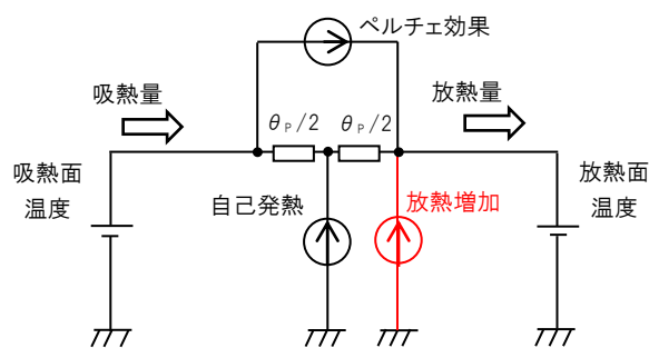
図5 ペルチェ素子の新しい熱等価回路
