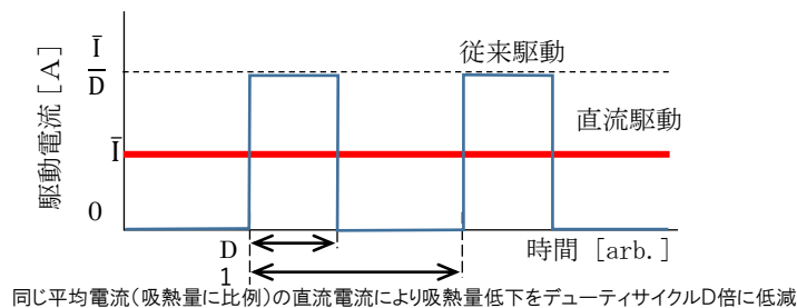
図2 ペルチェ素子の駆動電流波形
