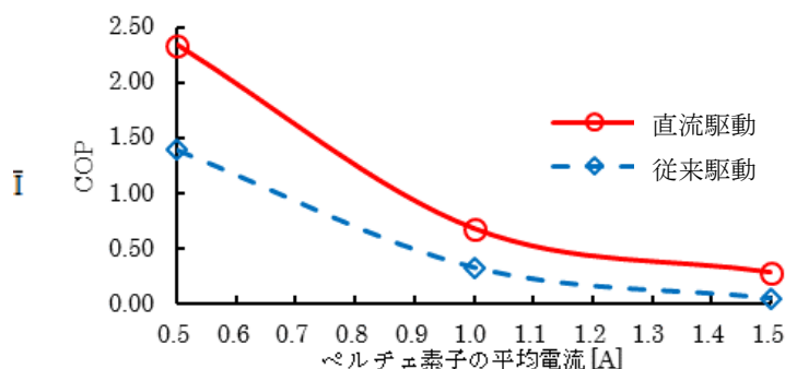
図4 成績係数 COP の特性
