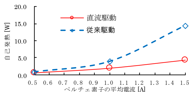
図3 ペルチェ素子の自己発熱の特性
