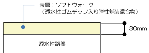
舗装断面例
