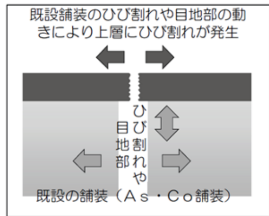
リフレクションクラック発生メカニズム
