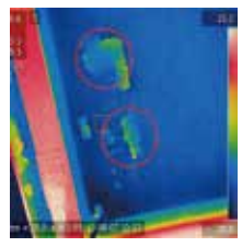
上) サーモグラフィカメラ 左) 熱画像による橋梁背面剥落部分抽出
