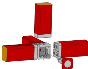
図2 JOSYの構造
