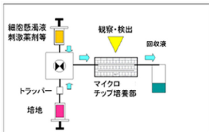
マイクロチップ灌流培養システム
