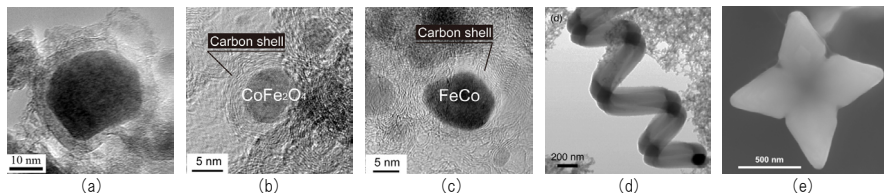
図 1 臨界流体中の自己集積化過程により形成されるナノ構造体。(a) フェロセン溶解二酸化炭素の光分解による鉄 (Fe) 内包カーボンナノ粒子の合成；(b) フェロセン・コバルトセン溶解ベンゼンの光分解による合金 (CoFe 2 O 4 ) 内包カーボンナノ粒子の合成；(c) フェロセン・コバルトセン溶解ベンゼンの光分解による合金 (FeCo) 内包カーボンナノ粒子の合成；(d) 銅錯体 (Cu(tbaoc) 2 ) 溶解ベンゼンの光分解によるカーボンナノコイルの合成；(e) フェロセン溶解エタノールの熱分解による非球形マグネタイト (Fe 3 O 4 ) ナノ粒子の合成
