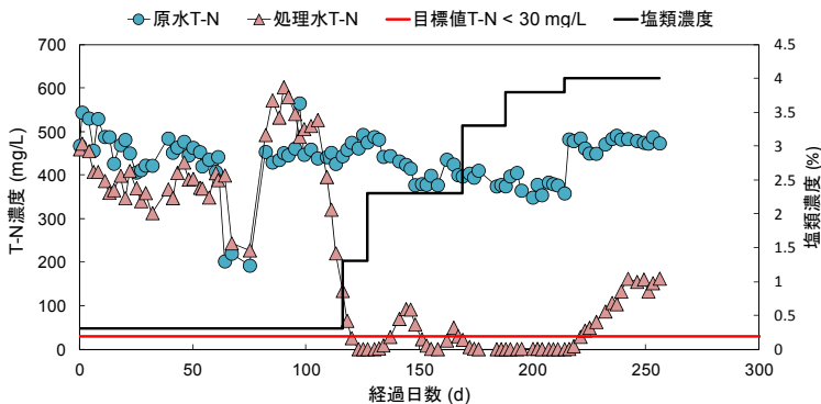
図1 連続処理運転での水質変化
