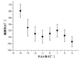
図3 ガラスイオン流路を通過した \text{Ar}^{3+} イオンビームのチルト角と観測角の関係
