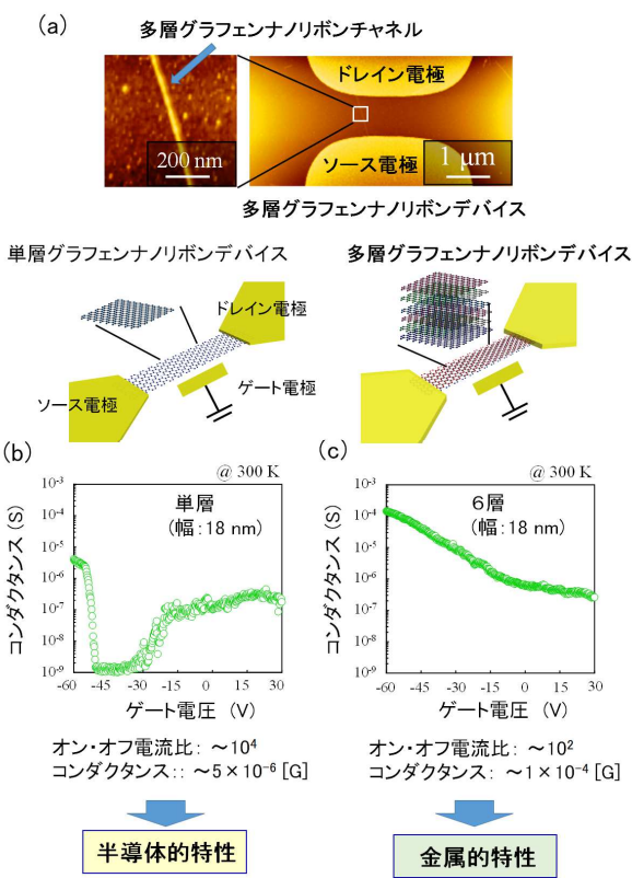
図3 (a)単一の多層グラフェンナリボンをチャンネルとした電界効果型トランジスタと、(b)単層グラフェンナリボンデバイスおよび、(c)多層グラフェンナリボンデバイスのキャリア輸送特性におけるゲート電圧依存性
