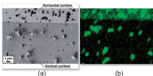
図 3 臨界点極近傍二酸化炭素中（31.0 °C）へのレーザー照射（波長 266 nm; 50,000 パルス）後に、基板上に生成された粒子。(a) 粒子の走査型電子顕微鏡像；(b) 元素分析（緑：炭素）。紫外線フォトンと二酸化炭素分子の相互作用により二酸化炭素分子が分解され、炭素粒子が生成される。
